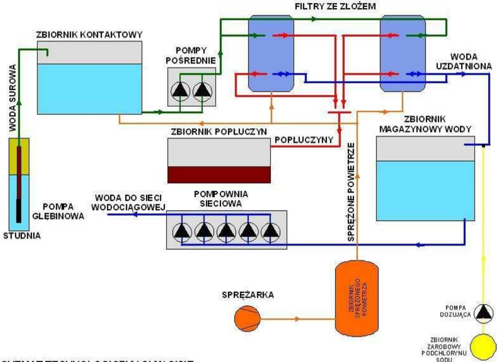
SCHEMAT TECHNOLOGICZNY SUW CISIE
